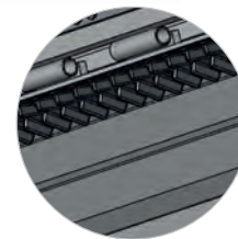
Прочный корпус с износостойкими пластинами в камере измельчения. Противорезающие пластины с термообработкой обеспечивают качественное измельчение
