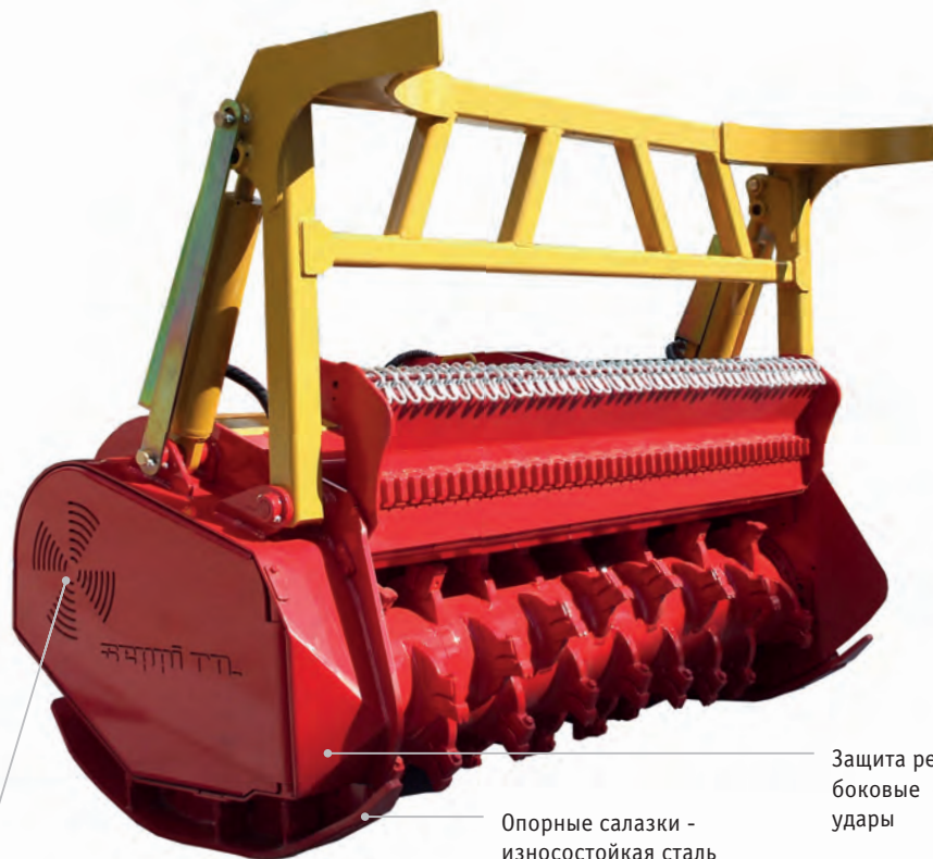
Рамка-толкатель защищает трактор и помогает в валке деревьев
