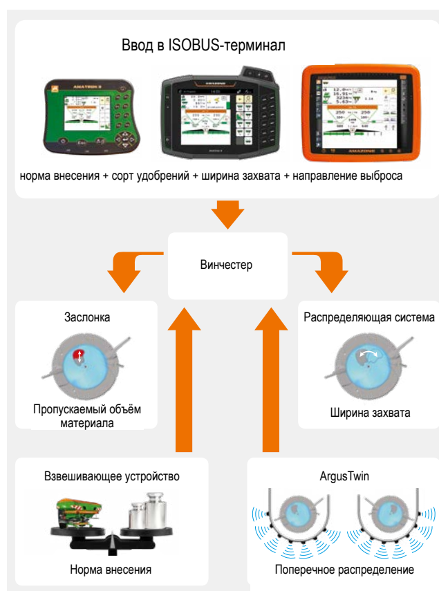
Концепция распределителей с ArgusTwin и системой взвешивания
