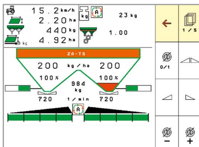
✓ Датчик опустошения бункера на ZA-TS
