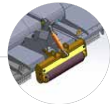
Je nach Anforderung wahlweise mit Stützwalze (Standard) oder drehbaren Stützrädern (Option)
